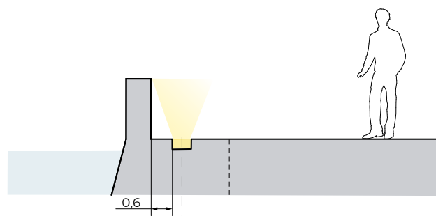
Светильник, встроенный в покрытие береговой зоны
